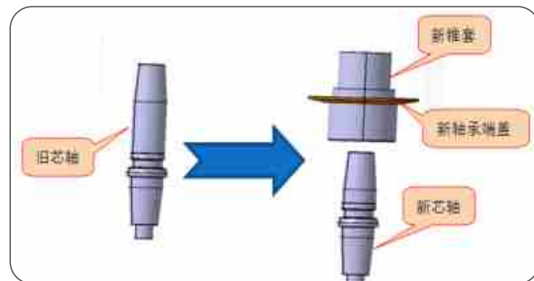
(图2) 芯轴结构优化
