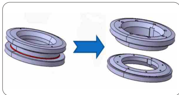
(图1) 轱环主辊模具由整体式改为分体式结构
